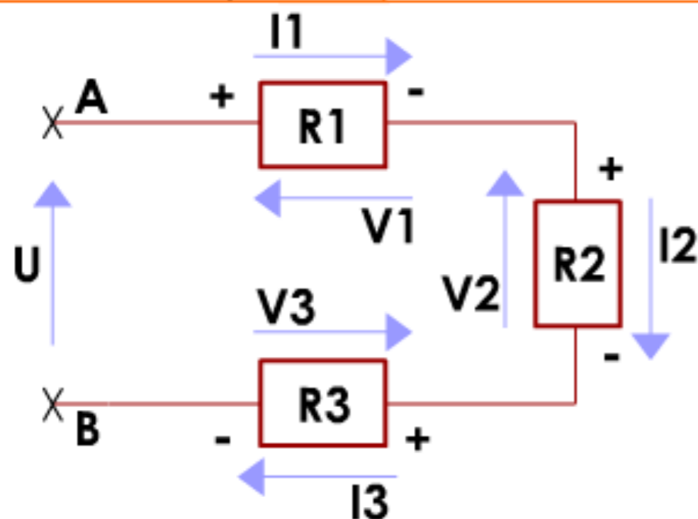
Schéma électrique
